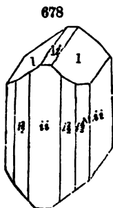
Schneeberg.
